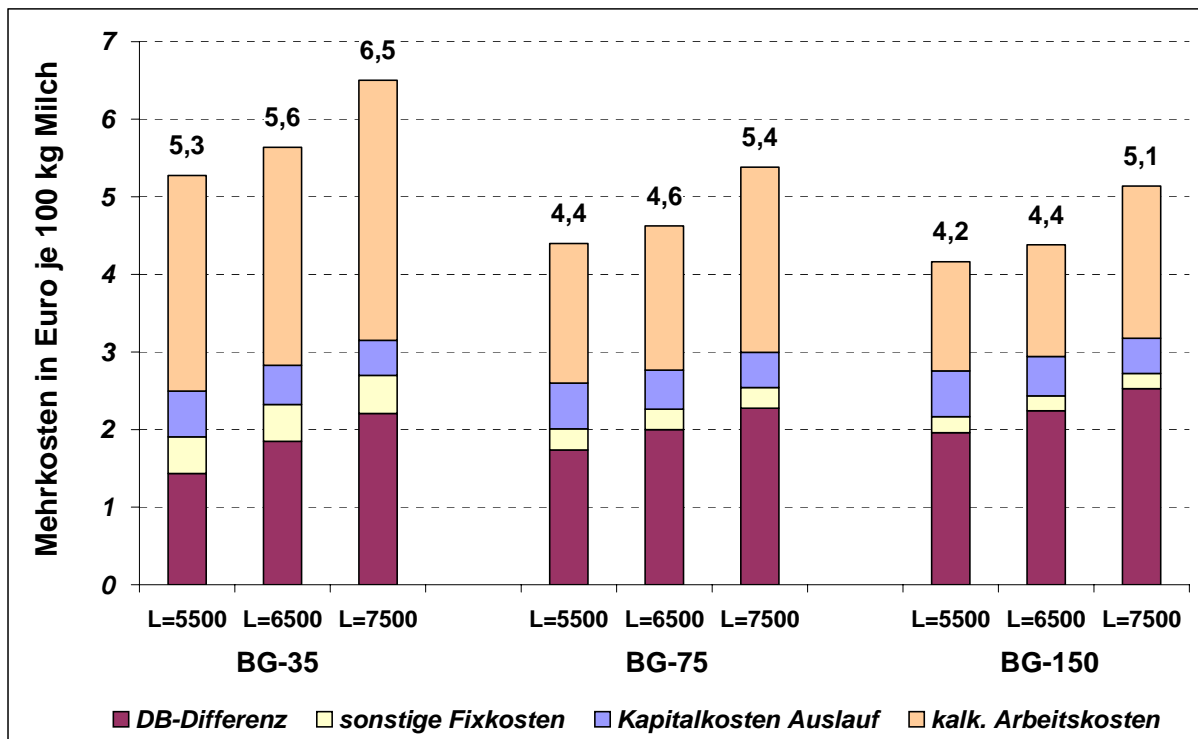
Abbildung 23: Mehrkosten je 100 kg Milch für den Biobetrieb gegenüber dem GLP-Betrieb bei Weiterführen der Anbindehaltung (Grünland)
