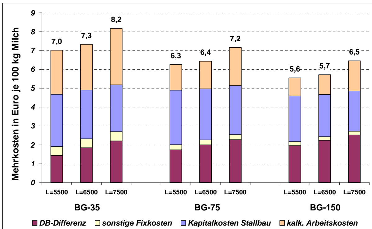
Abbildung 24: Mehrkosten je 100 kg Milch für den Biobetrieb gegenüber dem GLP-Betrieb bei Umstieg auf Laufstallhaltung (Grünland)
