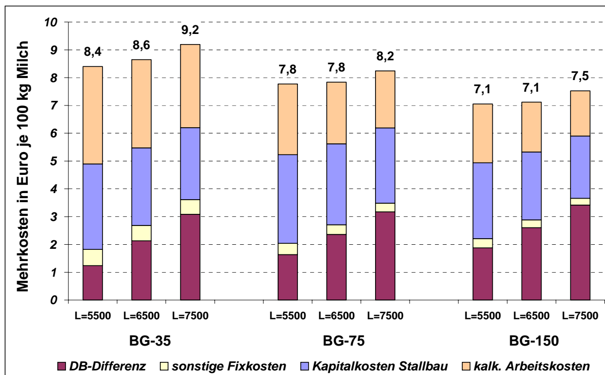
Abbildung 19: Mehrkosten je 100 kg Milch für den Biobetrieb gegenüber dem BV-Betrieb bei Umstieg auf Laufstallhaltung (Grünland)
