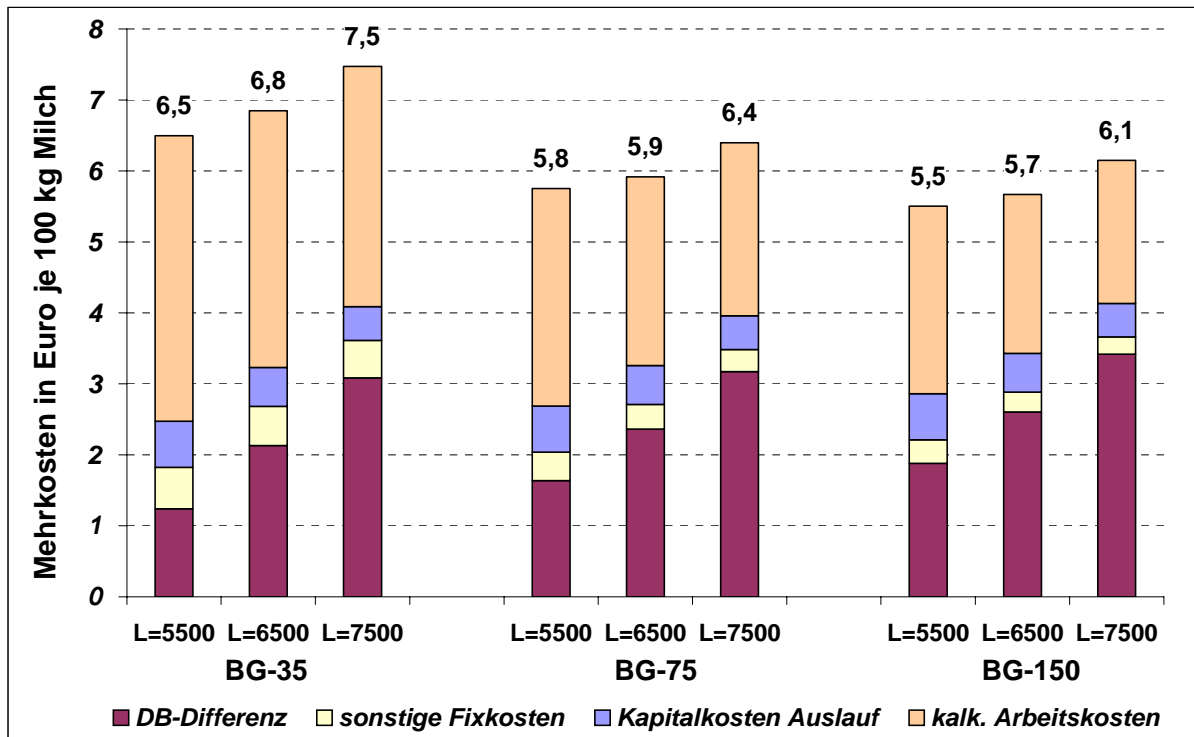
Abbildung 18: Mehrkosten je 100 kg Milch für den Biobetrieb gegenüber dem BV-Betrieb bei Weiterführen der Anbindehaltung (Grünland)
